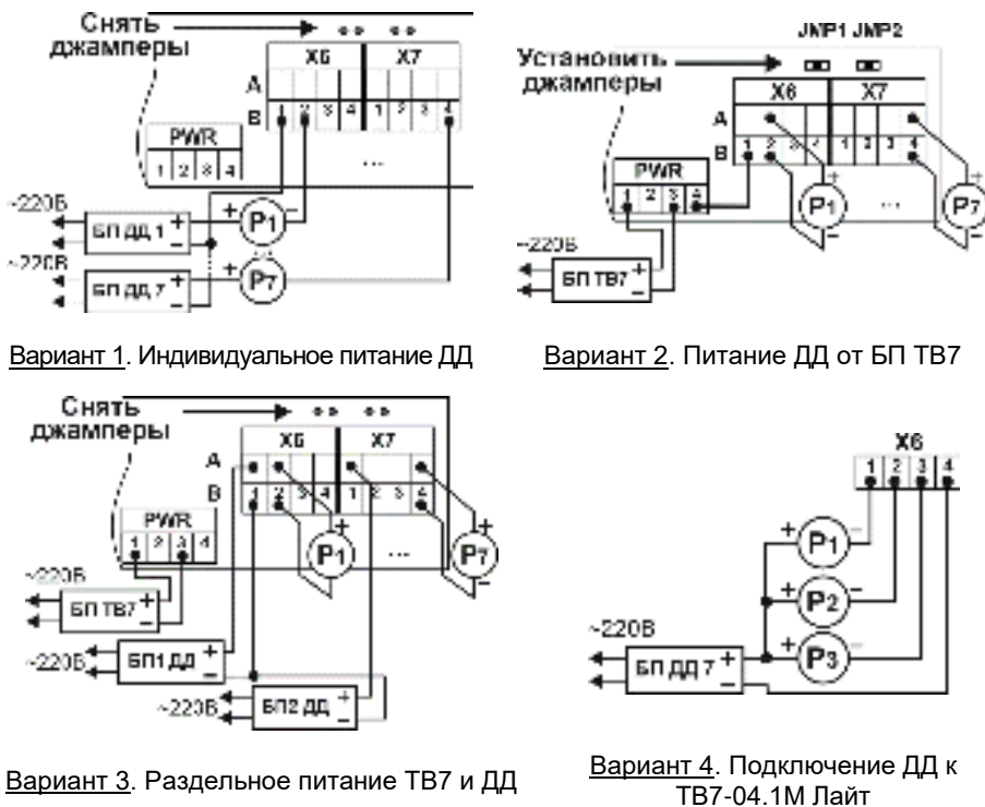
Рис. 4.6 – Примеры подключения датчиков давления к ТВ7
